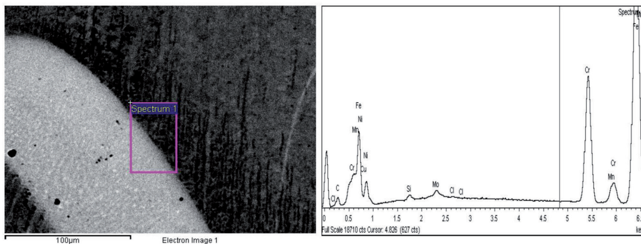
Figura 8: Micrografía y espectro SEM de la unión soldada sin atmósfera de argón en la zona interfase sin irradiar
