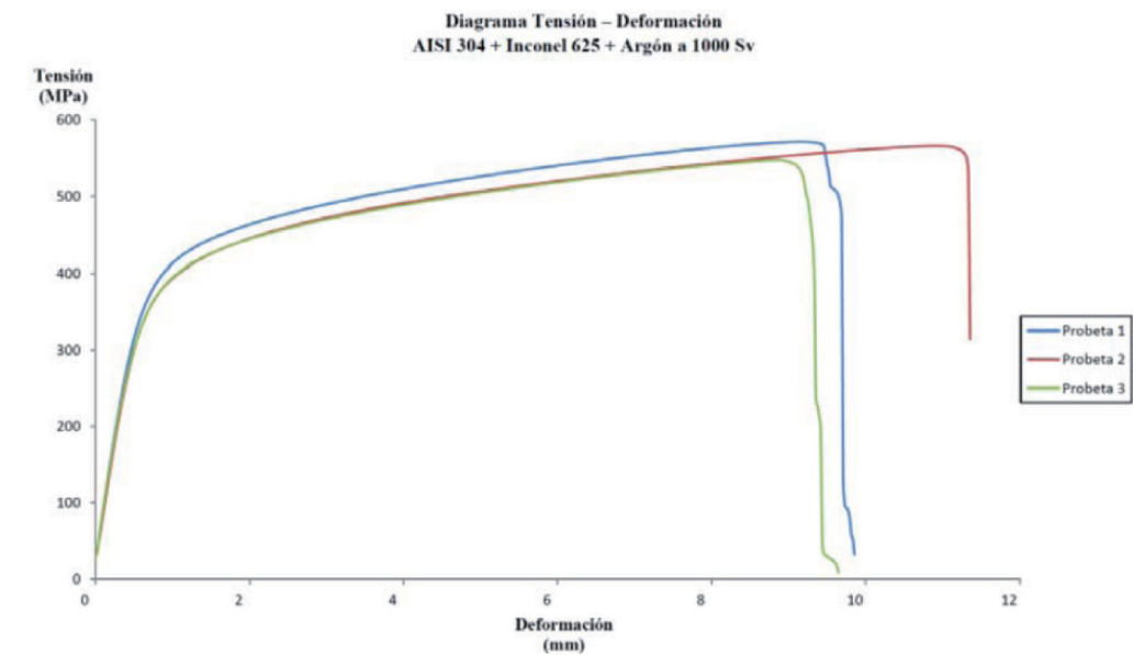
Gráfica 2: Ensayos de probetas 304 con aporte INCONEL 625 con cámara de atmósfera inerte de argón a tracción a 1000 Gy
