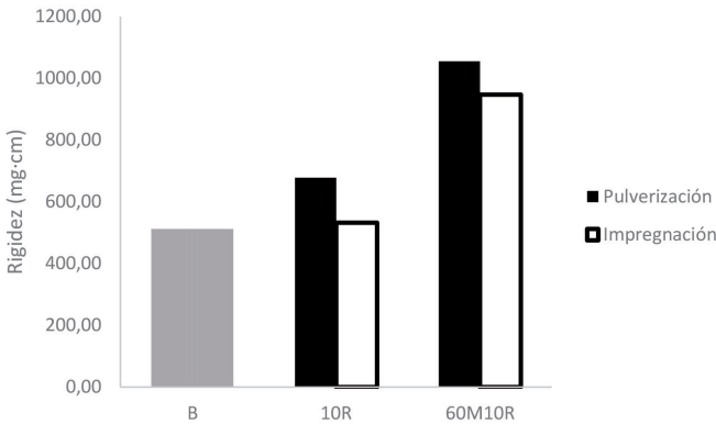
Figura 5: Representación de la rigidez obtenida en las muestras de 10 g/L de resina con y sin microcápsulas a 60 g/L de concentración aplicadas por impregnación y pulverización
