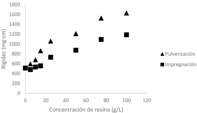
Figura 4: Gráfica de la rigidez a la flexión a diferentes concentraciones de resina en el tejido
