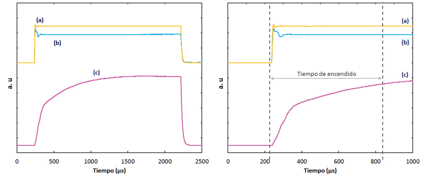
Fig. 3: Resultados característicos de funcionamiento del reactor de plasma: potencia incidente (a), potencia reflejada (b) y emisión luminosa visible (c)
