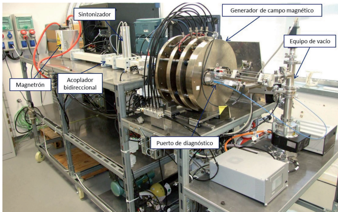
Fig. 2: Vista del reactor de plasma montado sobre el banco de pruebas donde son visibles los principales sistemas anteriormente descritos
