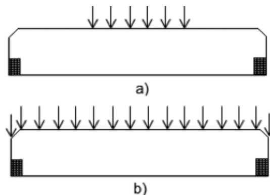
Fig. 2: Condiciones de carga crítica para la bovedilla de EPS
