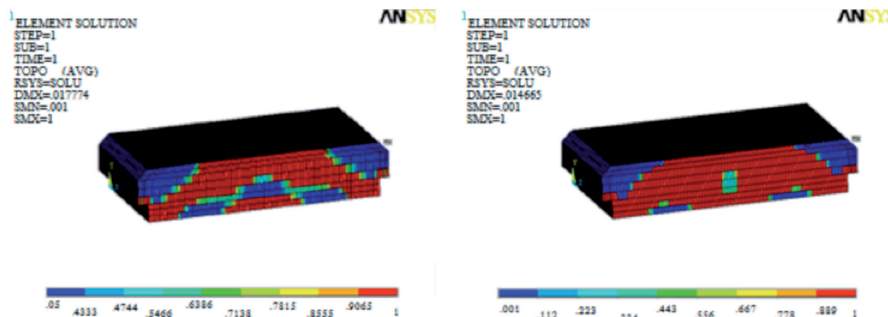
Fig. 8a) Segunda iteración del proceso de optimización b) Bovedilla de EPS optimizada topológicamente después de 12 iteraciones
