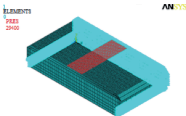
Fig. 7: Condiciones de carga y de frontera para la bovedilla
