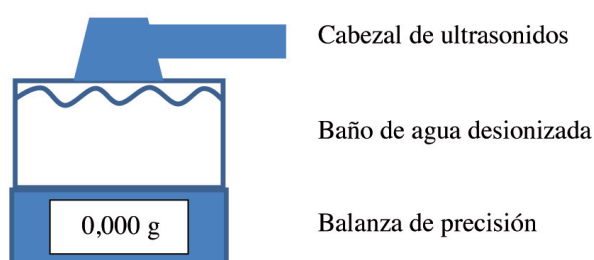
Fig. 2: Esquema de sistema de calibración de ultrasonidos, conforme a norma
